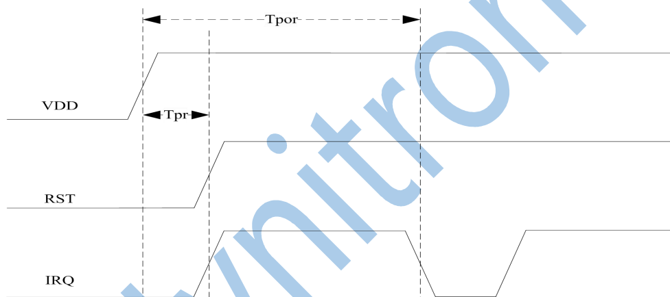
图 3. 上电时序图
