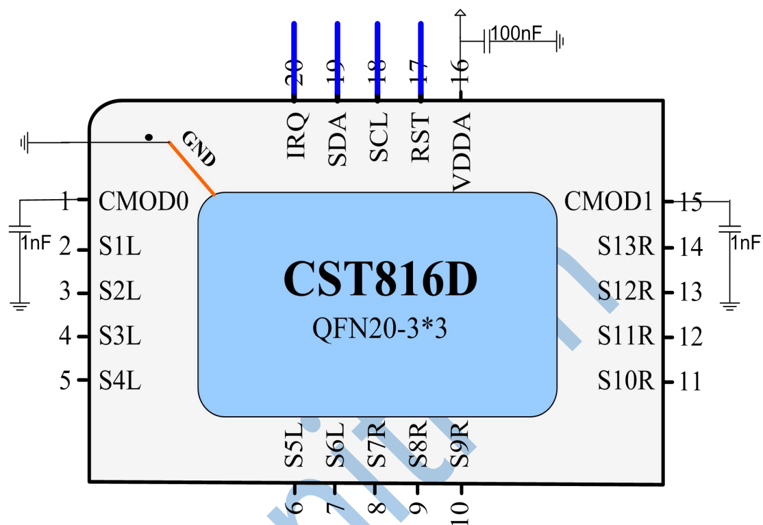
图 1. 参考电路图
