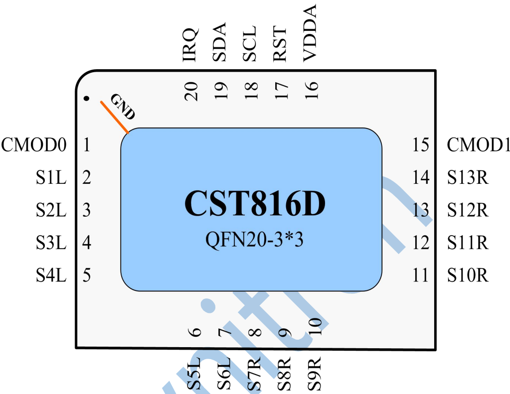
图 2. 引脚说明
