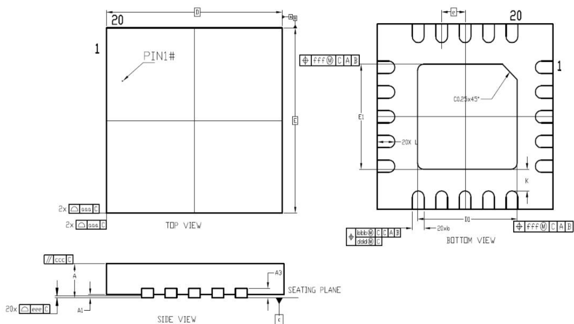
QFN20 外形图
